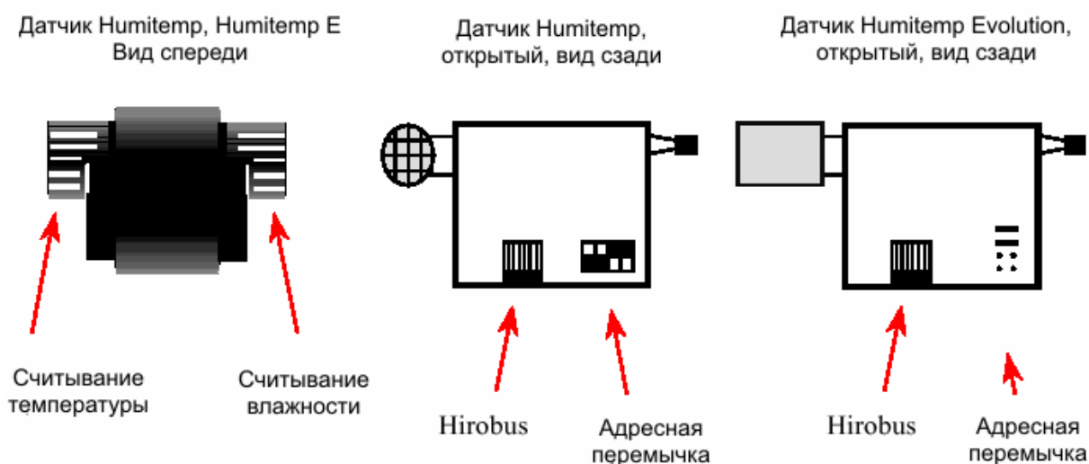
Рис. 13 Датчик Humitemp
