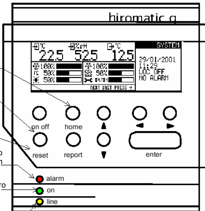
Рис.30 Модуль Hiromatic G с памятью E1G Eprom - вид спереди
